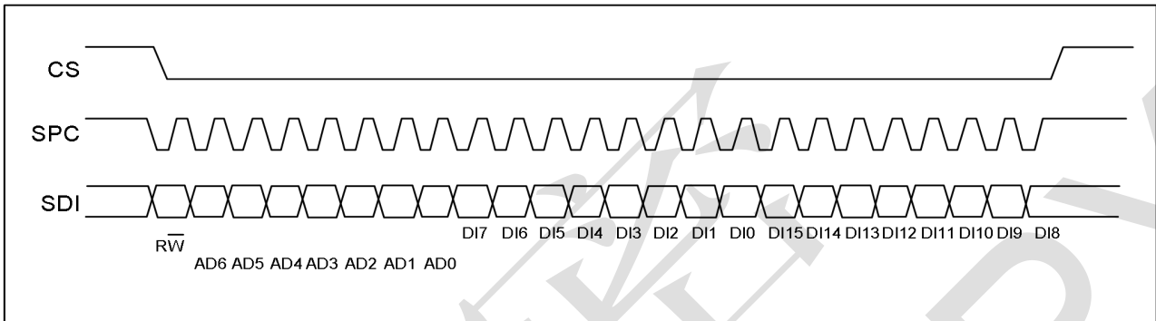
SPI多字节写协议 (2字节为例)
