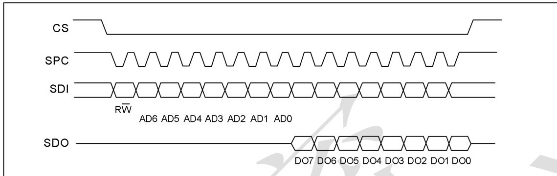
SPI读协议
