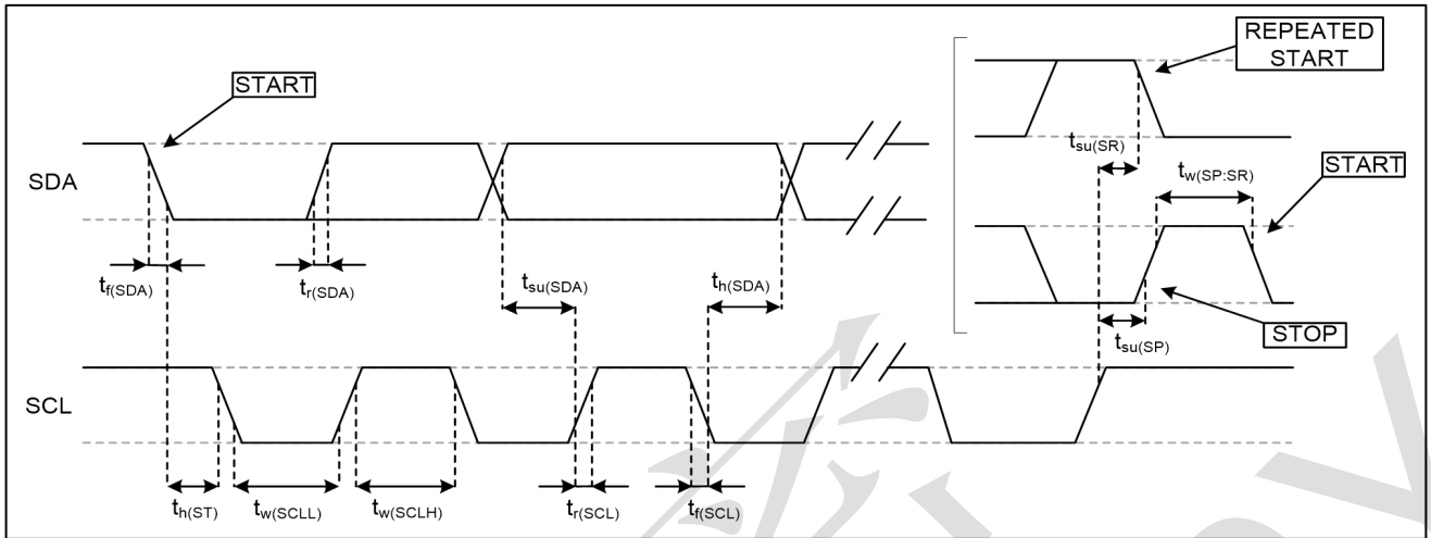
I²C 从设备时序图
