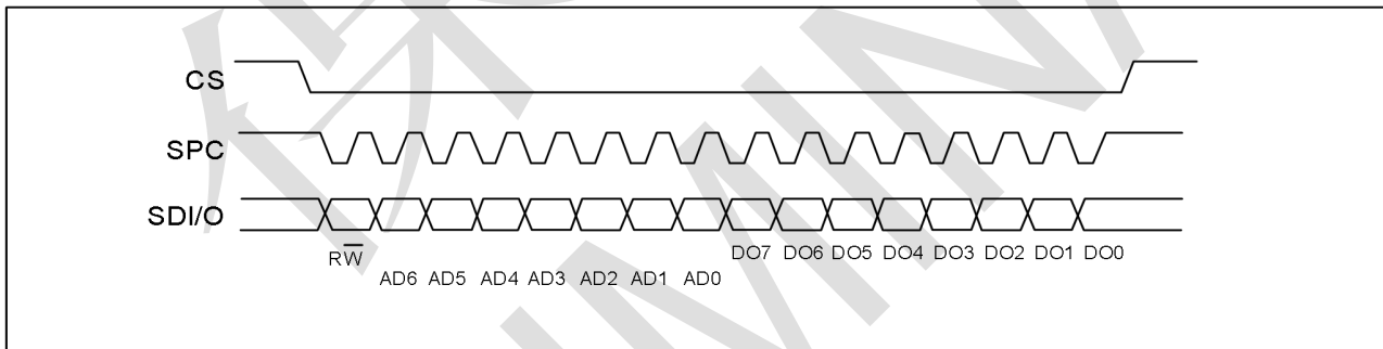
SPI 3线模式读协议
